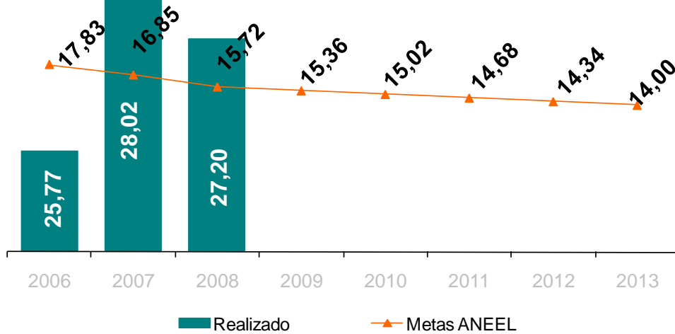
DEC AES Sul
